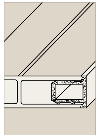
Abb. 6c: KAMMERPROFIL 16 für SDP 16
