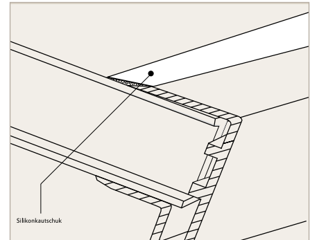
Abb. 5: Silikonkautschuk
