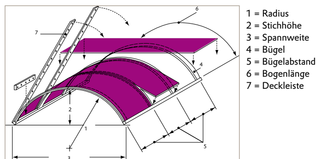
Abb. 3b: Prinzip kalt eingebogener Verlegung
