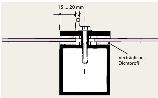
Abb. 2: Beispiel Metallträger
