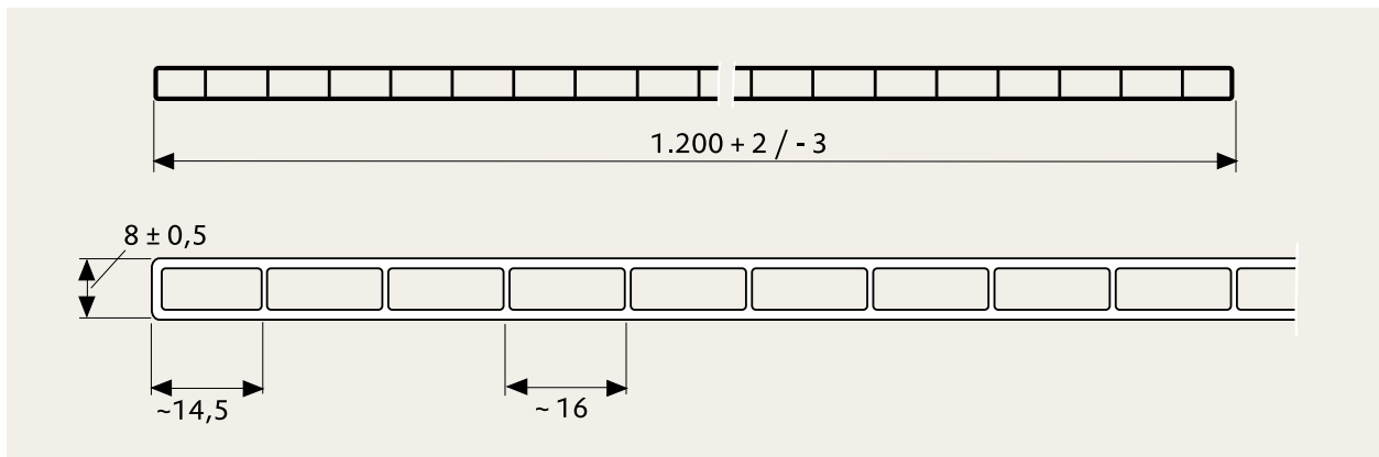
Querschnittbild der PLEXIGLAS RESIST® SDP 8 (Maße in mm)
