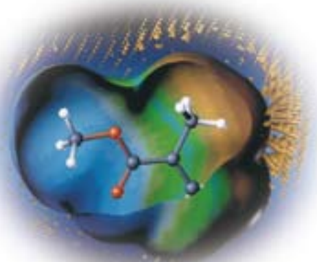
Monomer Methylmethacrylat, der kleinste Baustein von PLEXIGLAS®
